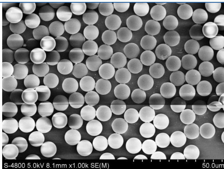
图1 SEM 形貌图/ SEM Image
